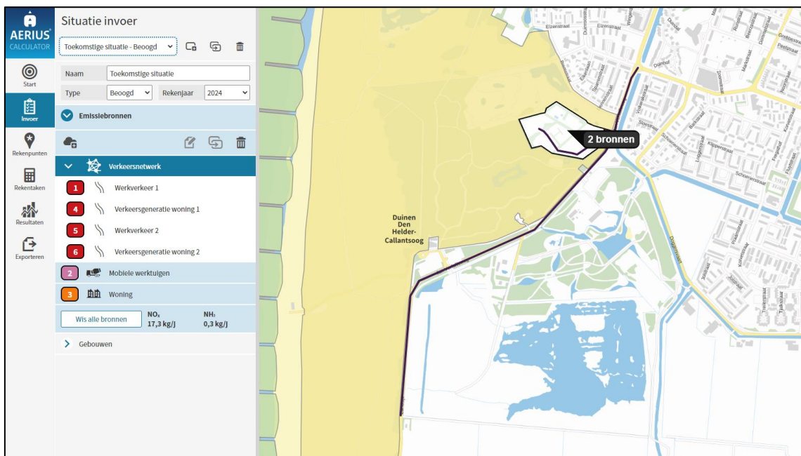
Afbeelding 4 - AERIUS-model aanlegfase
