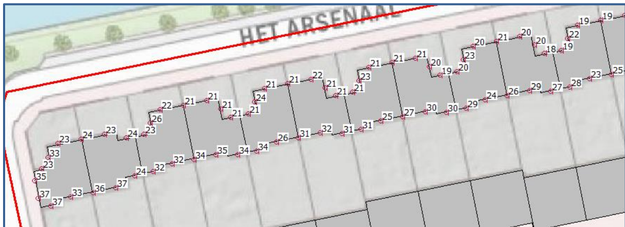
Afbeelding 5. Geluidbelastingen L_{den} (incl. aftrek art. 110g Wgh) Fazantenstraat Berekende maatgevende geluidbelastingen op een hoogte van 7,5 meter
