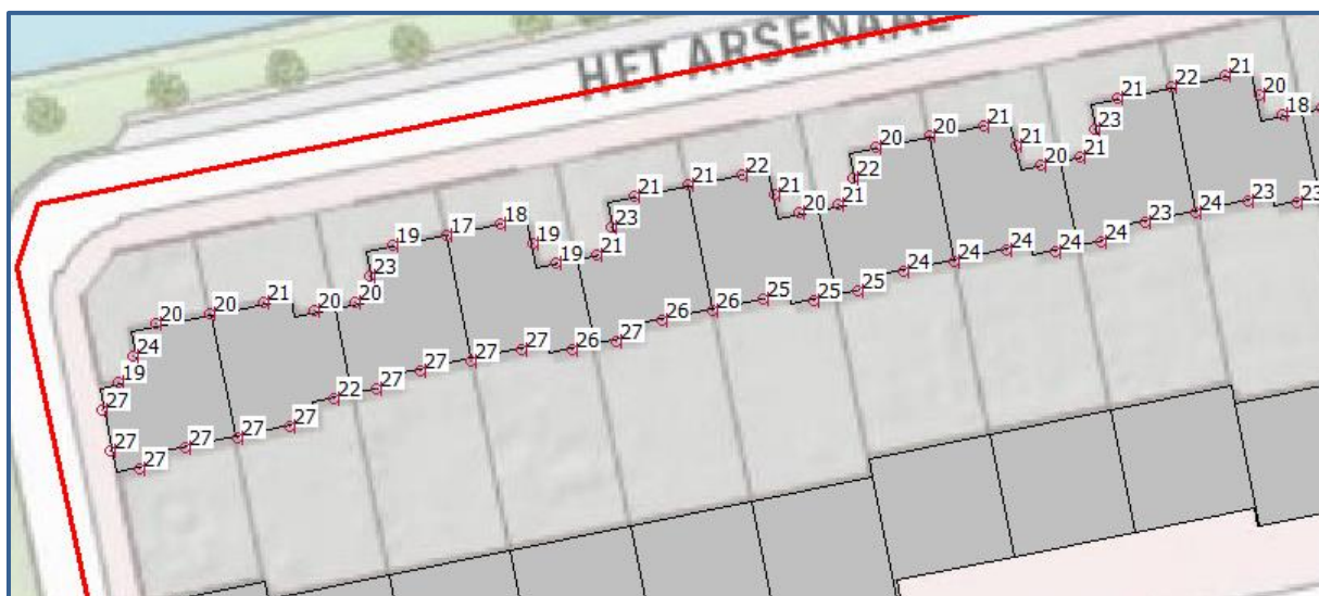
Afbeelding 7. Geluidbelastingen L_{den} (incl. aftrek art. 110g Wgh) Kievitstraat Berekende maatgevende geluidbelastingen op een hoogte van 7,5 meter
