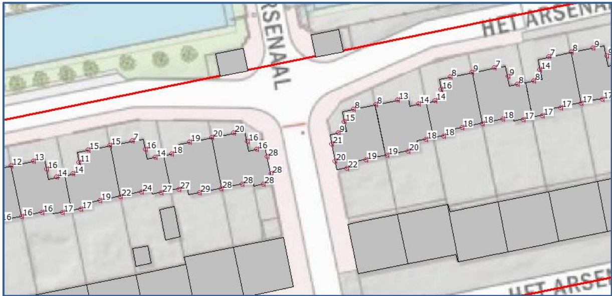
Afbeelding 8. Geluidbelastingen L_{den} (incl. aftrek art. 110g Wgh) Handelskade Berekende maatgevende geluidbelastingen op een hoogte van 7,5 meter
