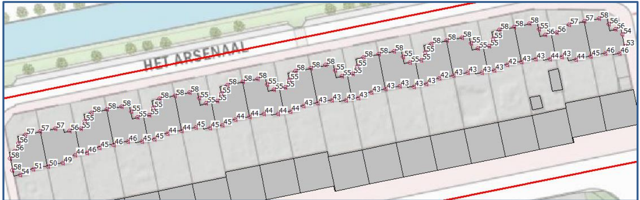
Afbeelding 9. Geluidbelastingen Lden (excl. aftrek art. 110g Wgh) cumulatief wegverkeer Berekende maatgevende geluidbelastingen op een hoogte van 7,5 meter
