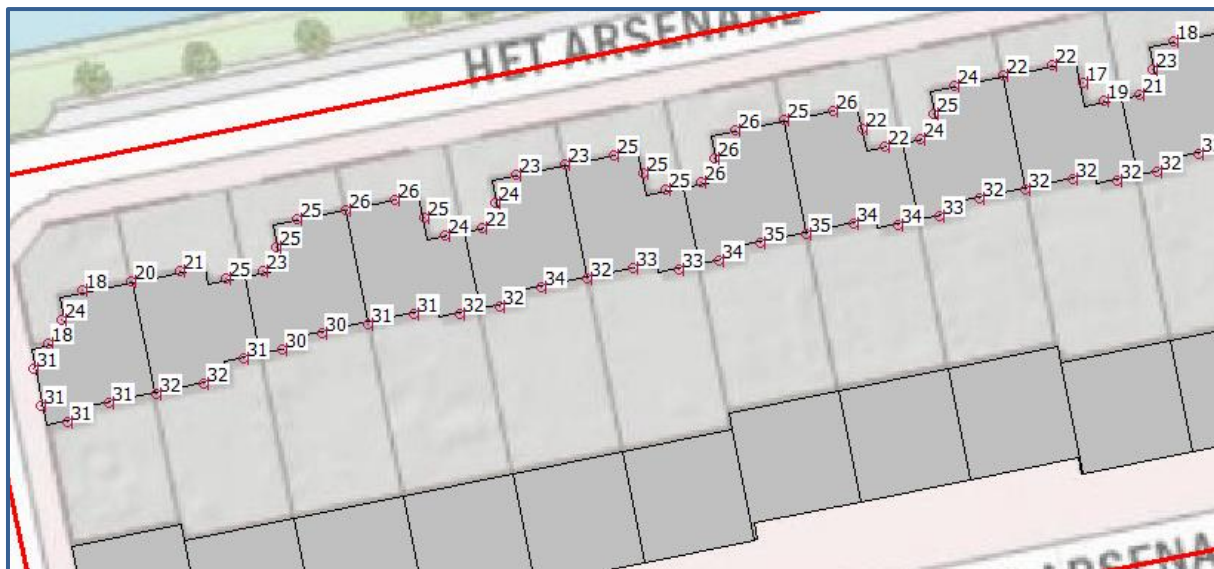
Afbeelding 6. Geluidbelastingen L_{den} (incl. aftrek art. 110g Wgh) Schootenweg Berekende maatgevende geluidbelastingen op een hoogte van 7,5 meter
