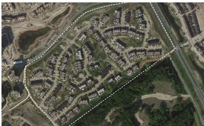
Zuiderduin, Almere 11.7 ha 229 woningen 20 woningen/ha
