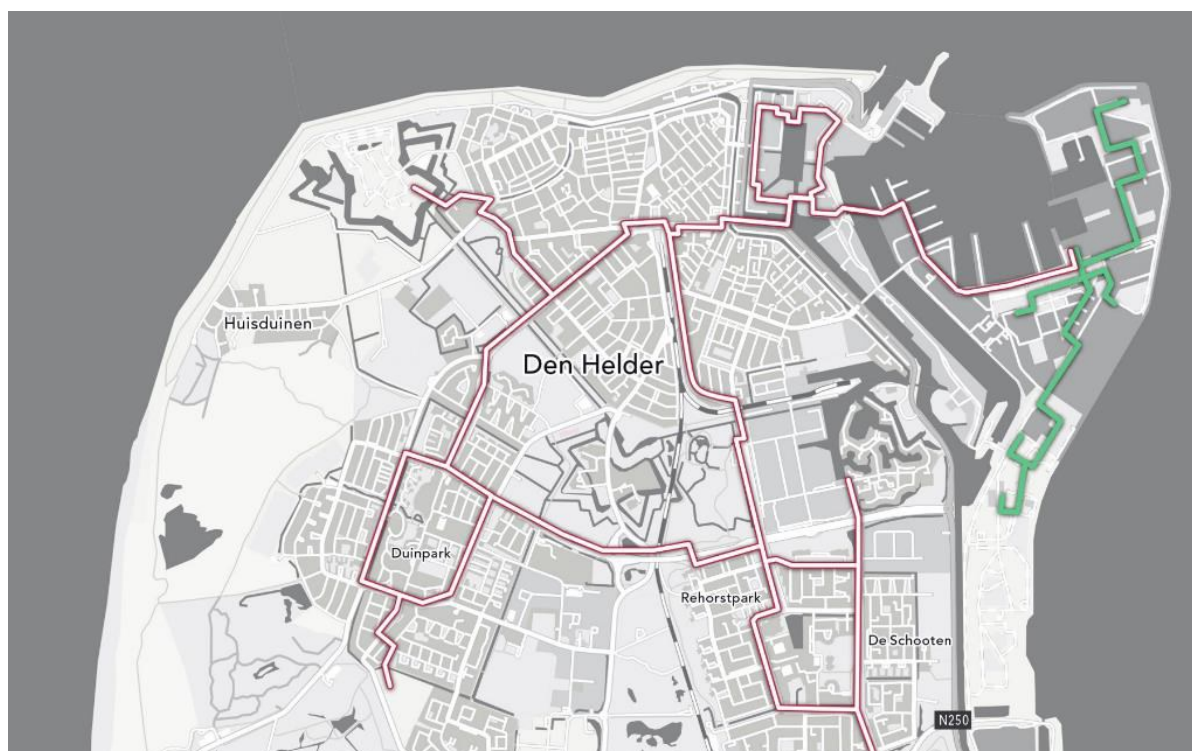
Figuur 1: Een mogelijk primair warmtenet in Den Helder. In groen weergegeven is het al bestaande warmtenet op het terrein van de Koninklijke Marine
