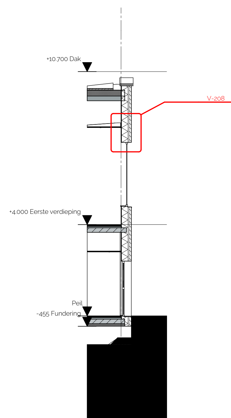
Doorsnede H-H 1
