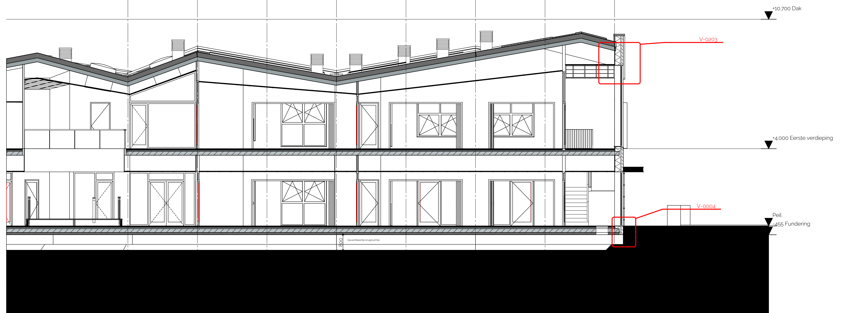
Doorsnede E-E
