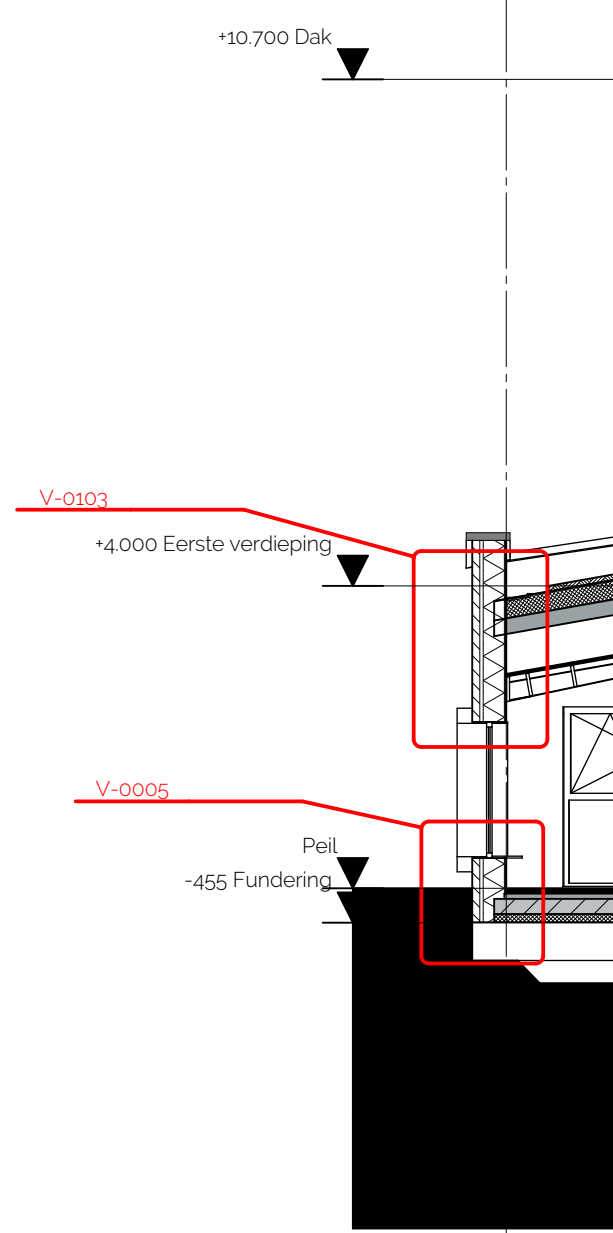
Doorsnede F-F A
