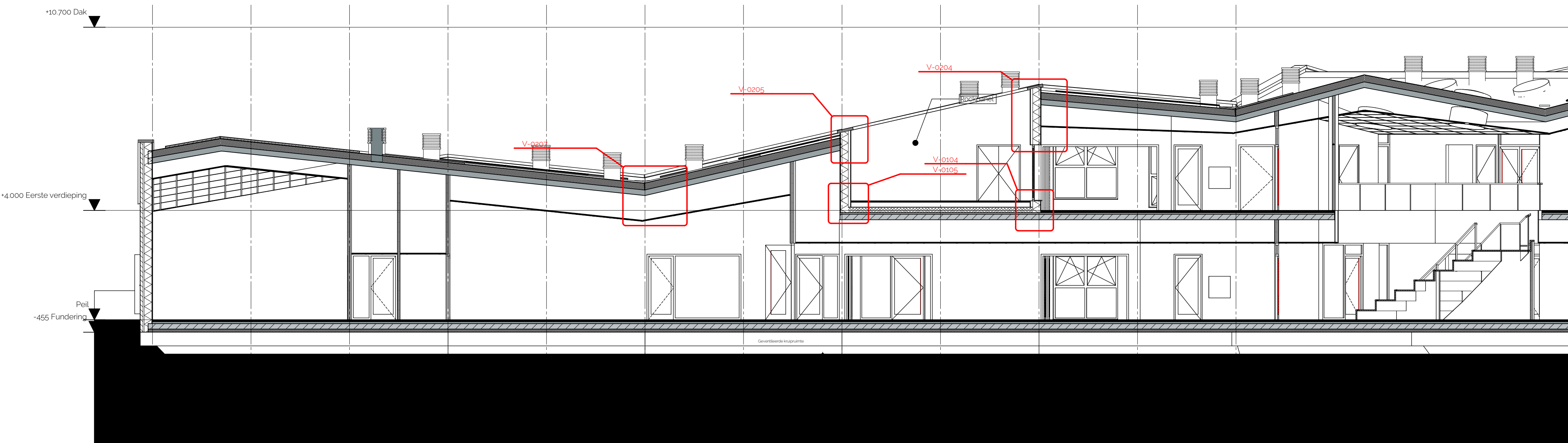
Doorsnede D-D
